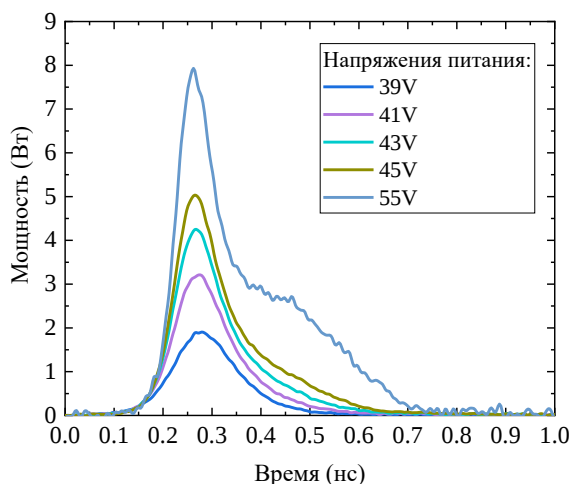
Рис.1. Динамика импульсов оптической мощности изготовленного модуля
