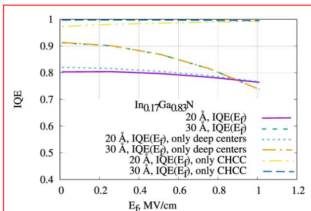
Рис.1. – Влияние различного типа процессов на ВКЭ приборов на InGaN/GaN.
