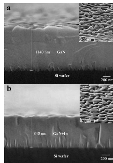
Рис.1. – SEM изображения кросс-секций и морфологии поверхности гетероструктур.
