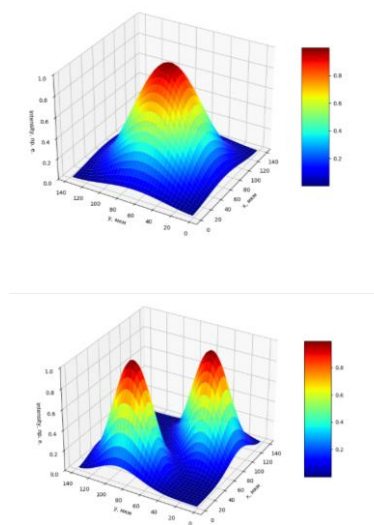
Рис.1. — Распределение интенсивности лазерного излучения в ближней зоне в излучающей апертуре 140 – 140 мкм полупроводникового лазера с резонатором на основе двумерного фотонного кристалла: фундаментальная мода, первая мода.
