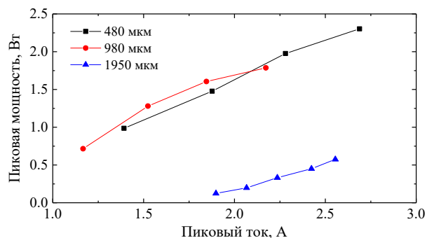
Рис.2. – ВтАХ образцов ЛТ разной длины
