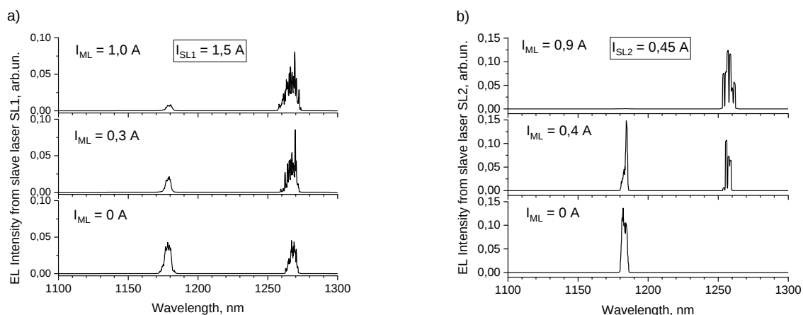
Рис.1. - Спектры излучения лазеров SL1 (а) и SL2 (б) при постоянном токе через каждый из них и различных уровнях оптической накачки (тока через ML). Ток инжекции лазера SL1 равен 1.5 А, а лазера SL2 - 0.45 А.
