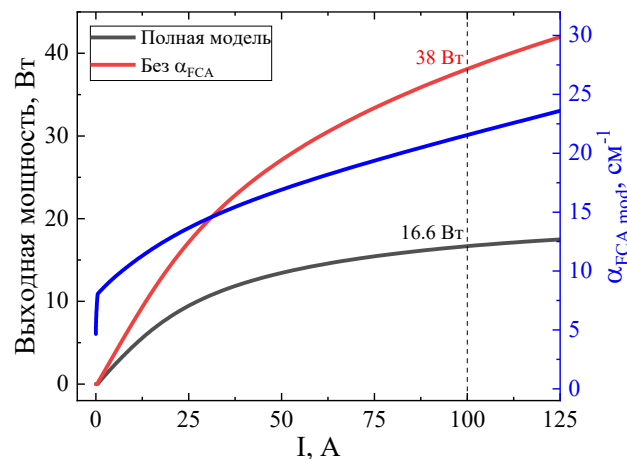
Рис.1. – Рассчитанные ВтАХ лазерных диодов в полной модели и модели с нулевыми потерями на свободных носителях заряда. Зависимость модальных оптических потерь от тока накачки (синяя линия).
