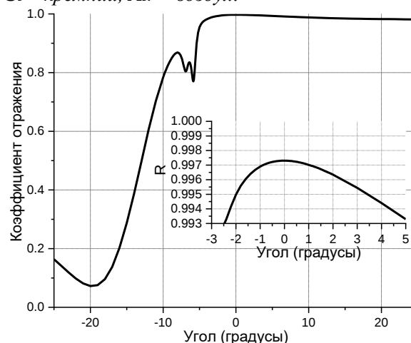
Рис.2. – Коэффициент отражения HCG для фундаментальной моды вертикально-излучающего лазера
