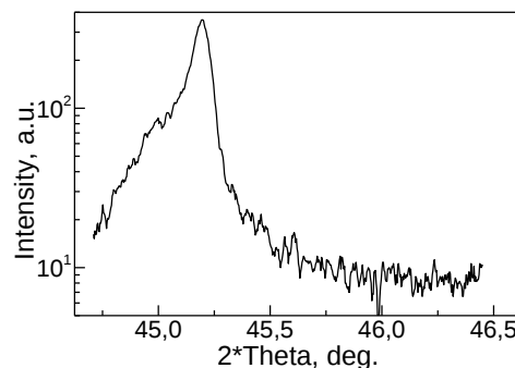
Рис. 1. – Участок рентгеновской дифрактограммы образца \text{ZnMnSe} в окрестности рефлекса \text{ZnSe} 220.
