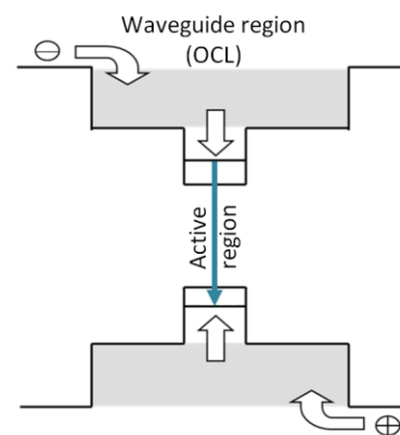
Рис. 1. Зонная диаграмма полупроводникового лазера с низкоразмерной активной областью
