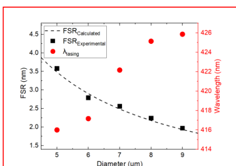
Рис. 2. – Экспериментальная (квадраты) и расчетная (прерывистая линия) зависимости FSR и спектрального положения лазерной линии (круги) от диаметра резонатора
