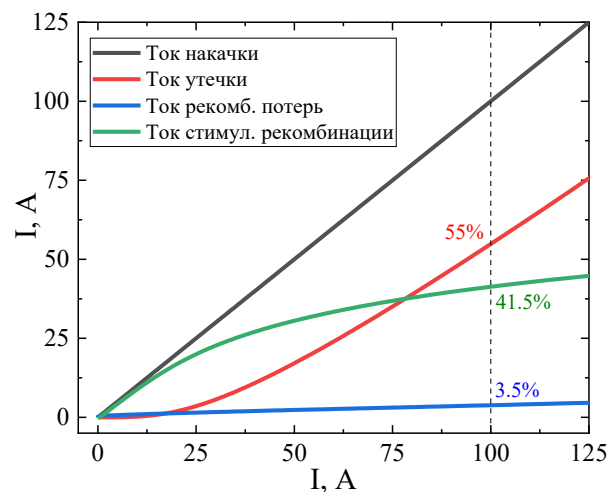
Рис.2. – Зависимость компонент тока (тока рекомбинационных потерь, тока утечки, тока стимулированной рекомбинации) от тока накачки.
