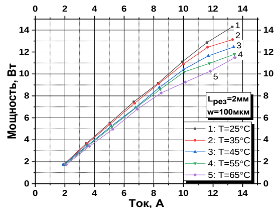
Рис. 1. – ВтАХ образца с шириной полоска 100мкм при разных температурах.
