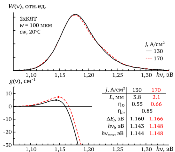
Рис.1.- Нормированные спектры спонтанного излучения, полученные при накачках 130 и 170 А/см 2 (вверху). Рассчитанные спектры модального усиления для соответствующих токов (внизу). Точками показаны положения максимумов усиления.
