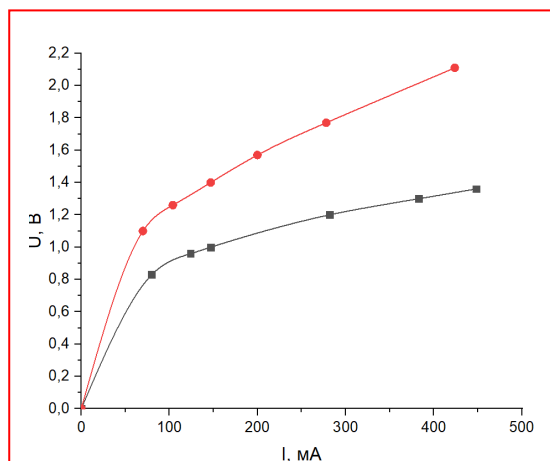
Рис.1. – Вольт-амперные характеристики образцов СЛД с использованием несплавного магнетронного (чёрный) и сплавного лазерного (красный) омических контактов.
