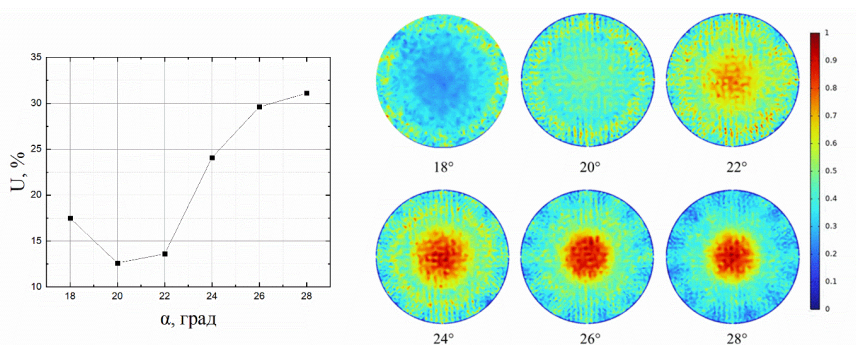
Рис.1 – Зависимость неоднородности распределения поглощенного излучения накачки U от угла ввода \alpha в активной области и распределения относительной поглощённой мощности излучения накачки при различных углах \alpha ввода излучения накачки.
