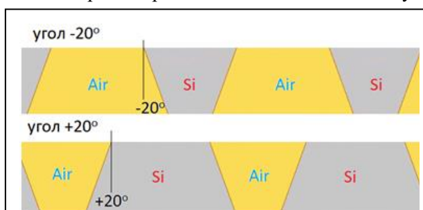
Рис.1. – Схематическое изображение формы штрихов HCG и наклона стенок канав для угла -20^\circ (сверху) и угла +20^\circ (снизу). Si – кремний, Air – воздух.
