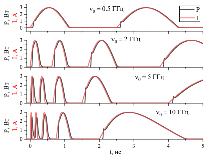
Рис. 1. – Модуляция сигнала лазерного диода с коротким высокодобротным резонатором при различной начальной частоте модуляции.
