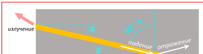
Рис.1. – Схематическое изображение суперлюминесцентного диода со скользящим полосковым волноводом.
