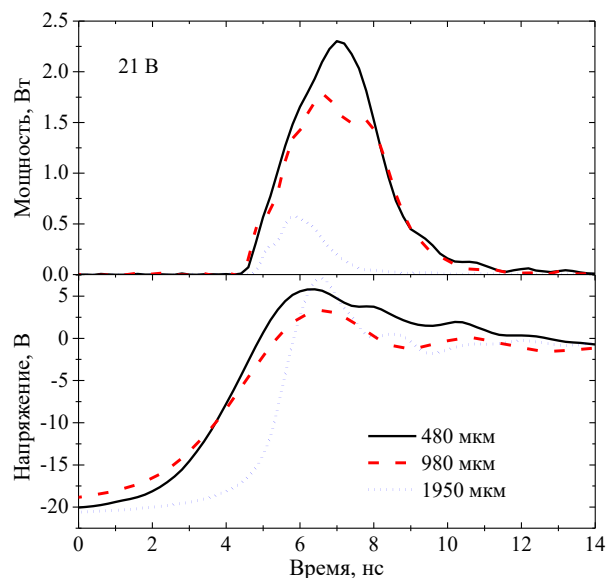
Рис.1. – Динамика мощности (а) и напряжения на конденсаторе (б) при напряжении питания 21 В
