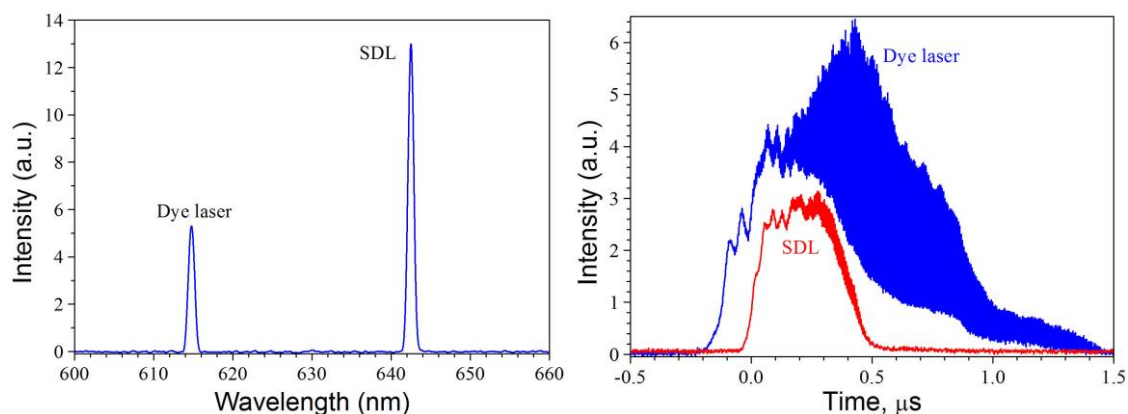
Рис. 2. – Спектр генерации (слева) и осциллограммы импульсов (справа) лазера на красителе и ПДЛ.
