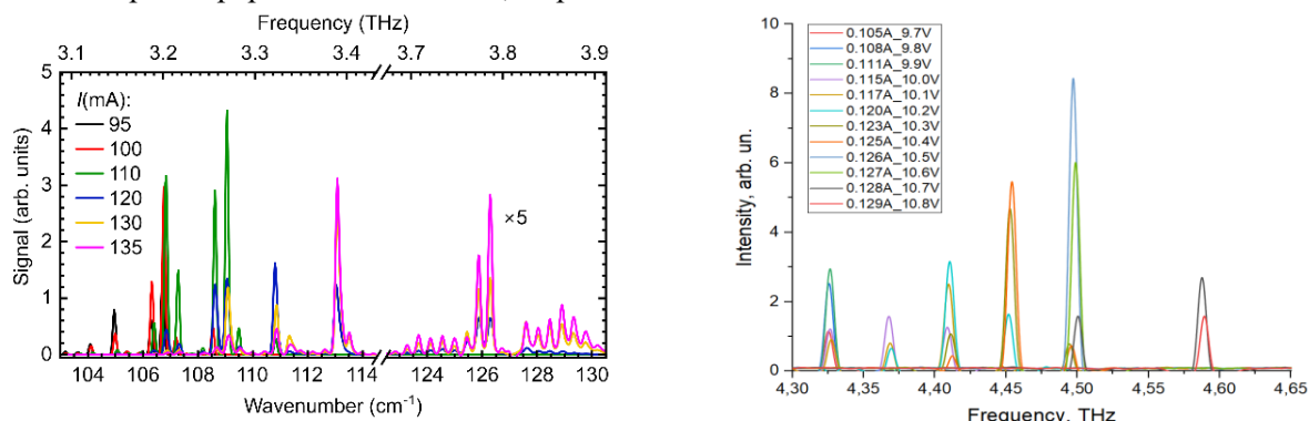
Рис. 1. – Спектры генерации непрерывных МПЭ ТГц ККЛ (слева) и МОСГЭ ТГц ККЛ (справа).
