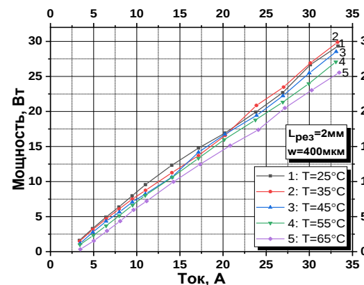
Рис. 2. – ВтАХ образца с шириной полоска 400мкм при разных температурах.
