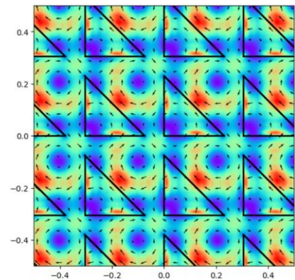
Рис.1. – Распределение электрического поля (стрелки) и интенсивности (цвет) для фотонного кристалла, сформированного равнобедренными прямоугольными треугольниками, черные сплошные линии демонстрируют границы отверстий.
