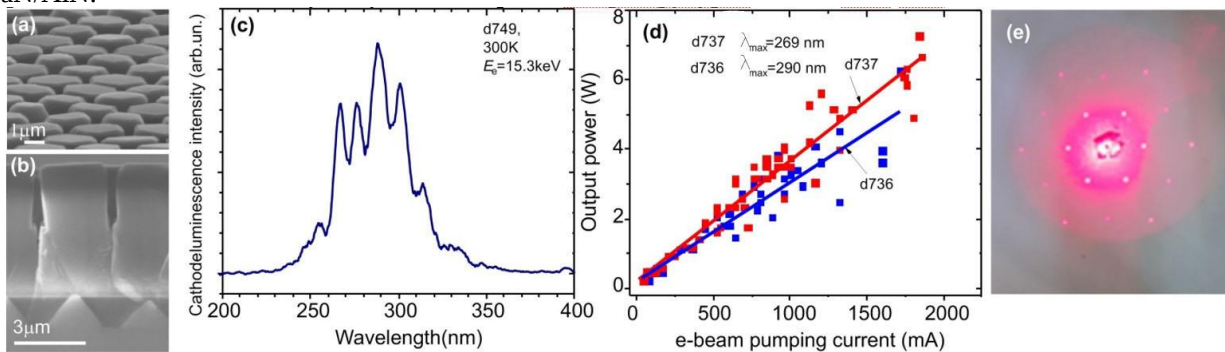
Рис.1. - Изображения поверхности (а) и поперечного сечения (б) AlN микрорезонаторов с множественными КЯ GaN/AlN, полученные с помощью растрового электронного микроскопа. Спектр катодолуминесценции (с) и зависимости выходной импульсной оптической мощности от электронного тока накачки (д) для различных микрорезонаторных структур с МКЯ GaN/AlN. (е) Интерференционная картина, формирующаяся при нормальном отражении лазерного луча от поверхности структуры с микрорезонаторами.
